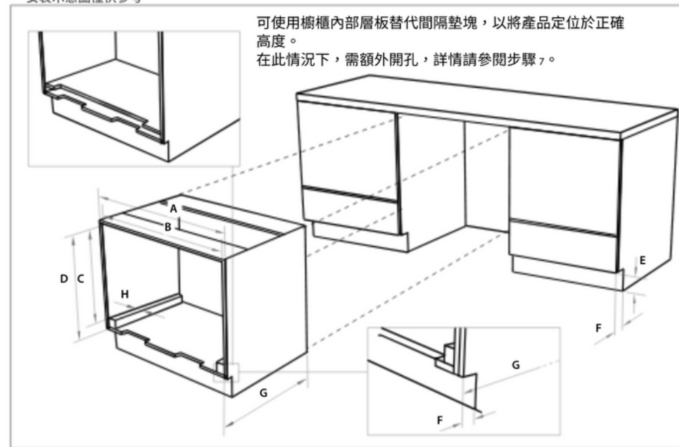
櫥櫃尺寸(mm)
