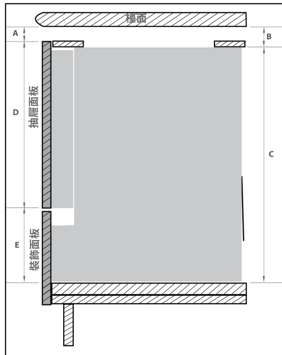
側面圖
