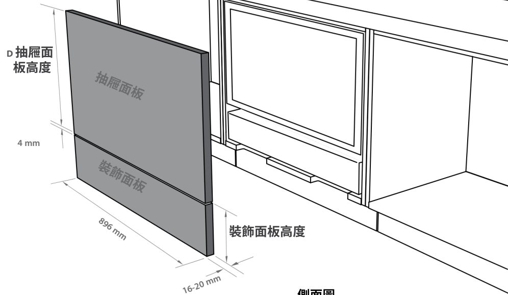
側面圖
