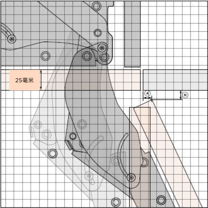
25 毫米覆蓋式門板 A 門邊距櫥櫃側邊距離：14 毫米 B 門角與相鄰櫥櫃之間的間隙：12 毫米 注意：覆蓋式面板的寬度需相應調整。
