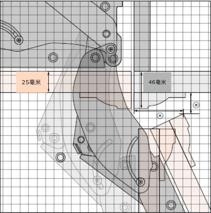
25 毫米門板，搭配 19 毫米框架 A 門邊距櫥櫃側邊距離：60 毫米 B 門角與相鄰櫥櫃之間的間隙：26 毫米
