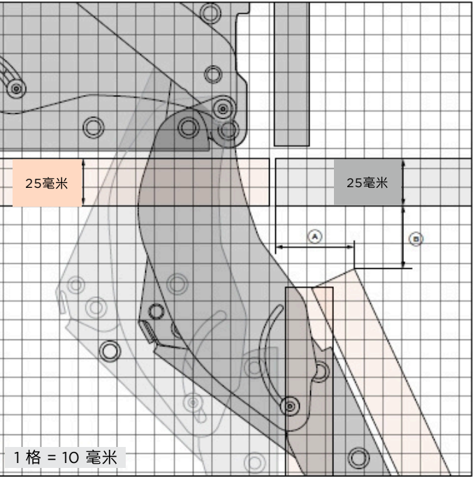
25 毫米門板 A 門邊距櫥櫃側邊距離：42 毫米 B 門角與相鄰櫥櫃之間的間隙：34 毫米
