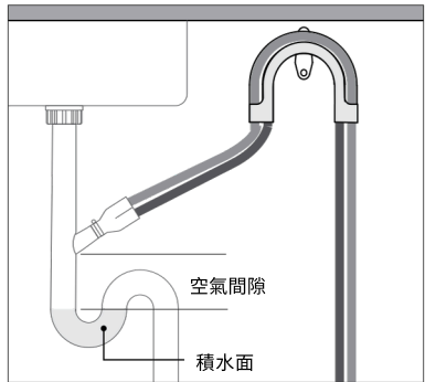
細部圖－水龍頭安裝
