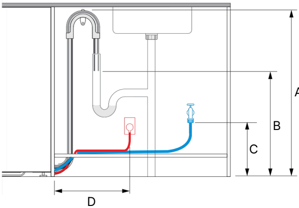
正面剖面圖－管路安裝
