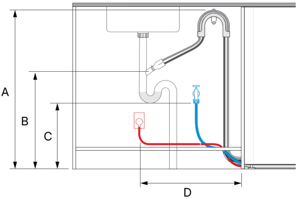
正面剖面圖－水龍頭安裝
