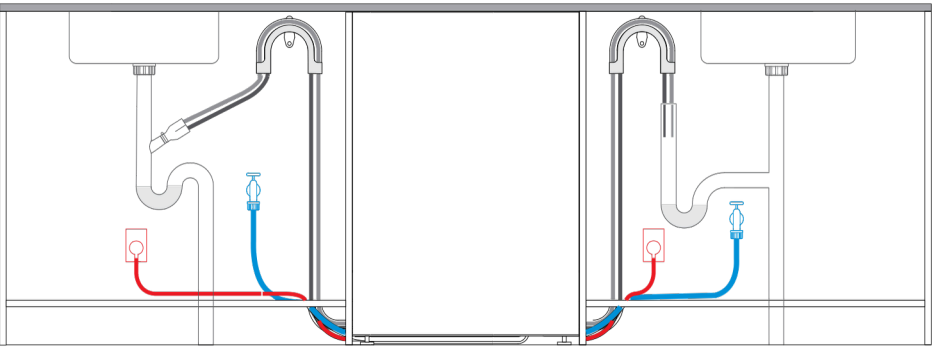
正面剖面圖－踢腳板內的管路配置
